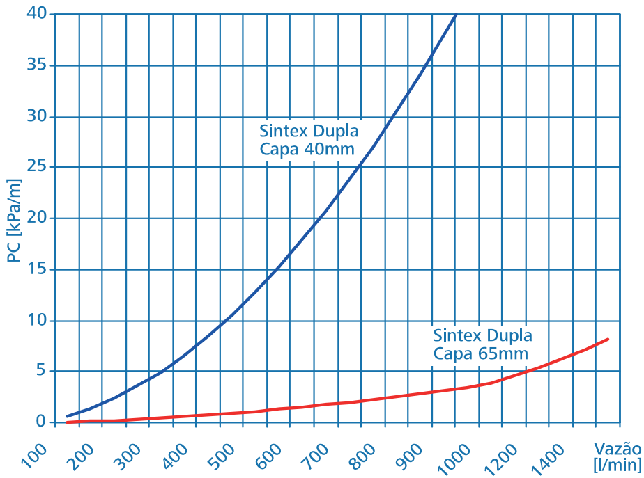
Gráfico de perda de carga
